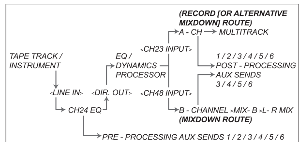
Fig. 4.3: Post EQ channel insert
