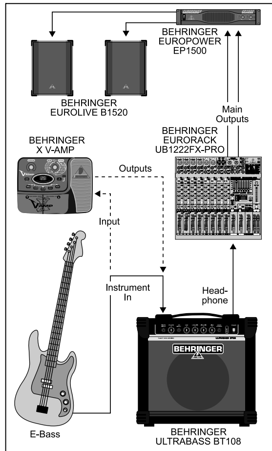
Fig. 2.2: Live setup
